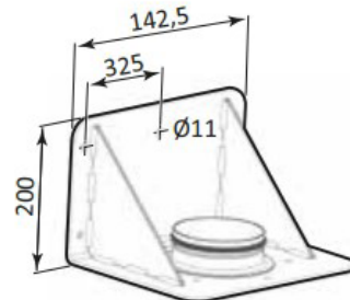
Seinäkannake
