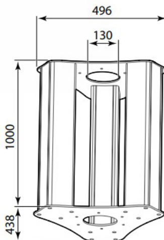
Kattokannake
