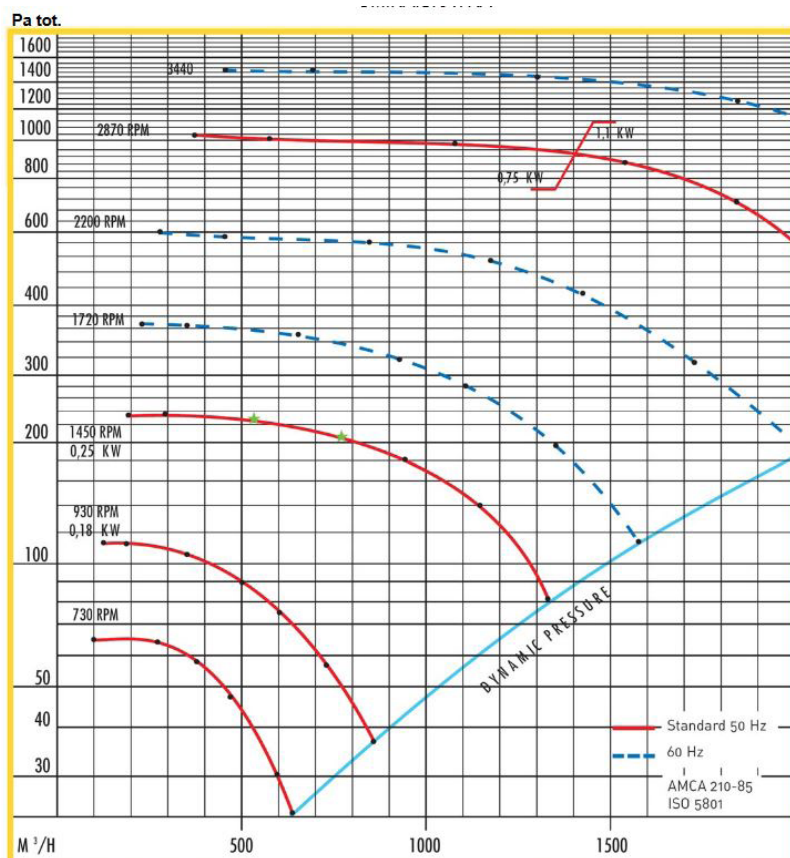
P-20 ominaiskäyrä
