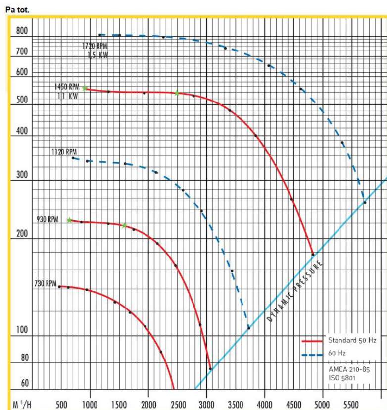
P-30 ominaiskäyrä
