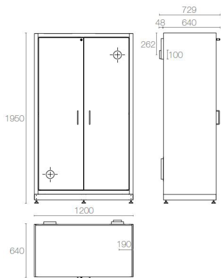
AC 1200 S
