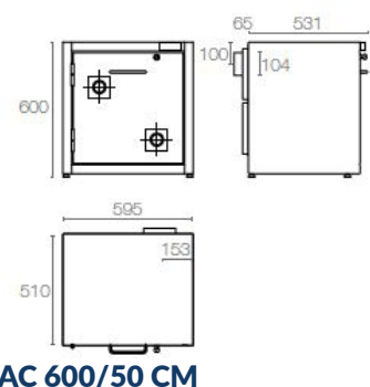
AC 600/50 CM
