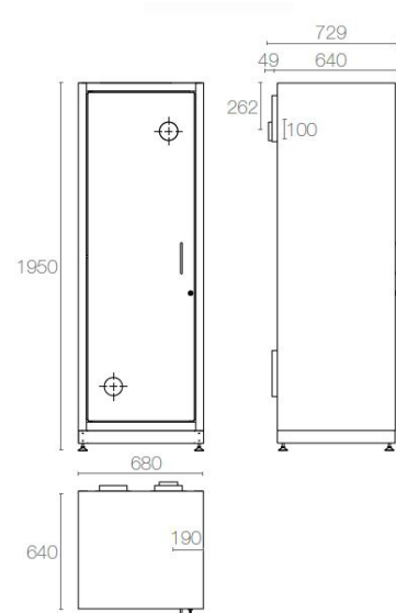
AC 600 S
