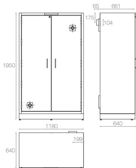
AC 1200 CM
