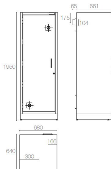
AC 600 CM
