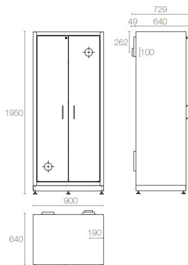
AC 900 S
